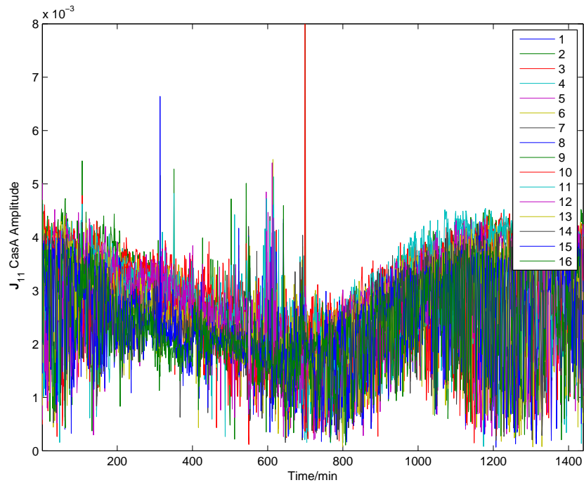
CasA G_{11}
